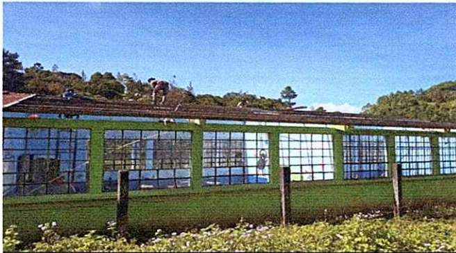
Foto 1: Desinstalacion lámina acanalada en mal estado por lamina troquelada.
